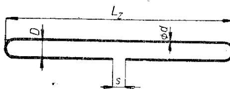
Obr. 58. Skládaný dipól
