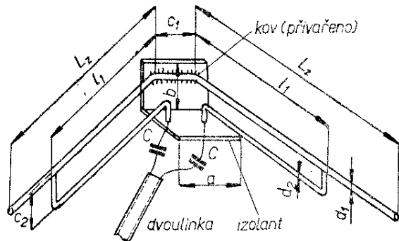
Obr. 49. Anténa pro I. televizní pásmo
