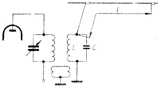
Obr. 80. Připojení antény typu Fuchs ke koncovému stupni vysílače
