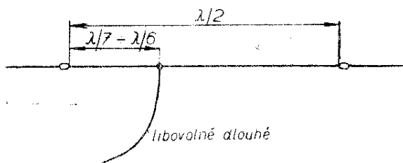
Obr. 81. Anténa typu Windom
