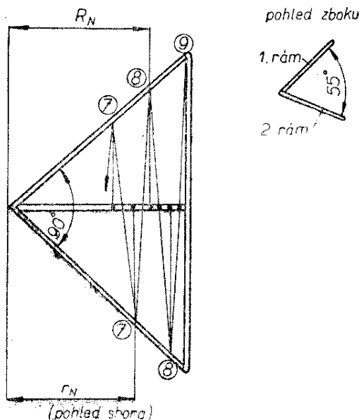
Obr. 76. Logaritmicko-periodická anténa
