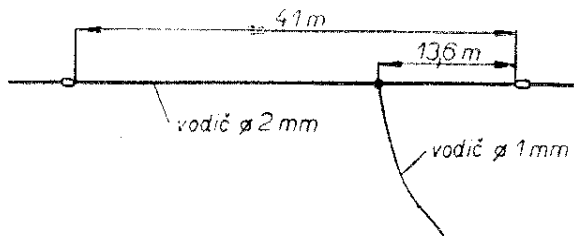
Obr. 83. Anténa VSIAA
