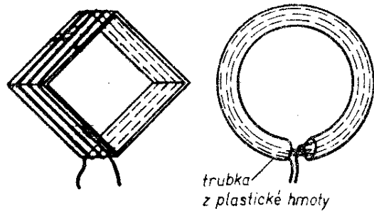
Obr. 24. Rámová anténa
