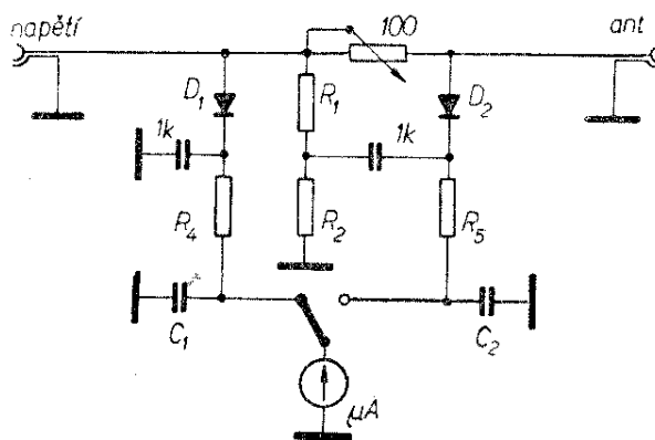
Obr. 133. „Matchmaker“
