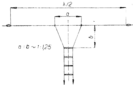
Obr. 19. Transformace Delta
