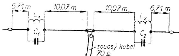
Obr. 111. Anténa W3DZZ
