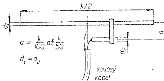
Obr. 20. Transformace Gamma
