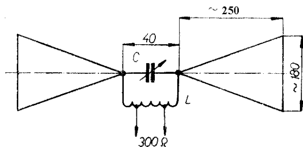
Obr. 50. Náhradková anténa pro III. televizní pásmo
