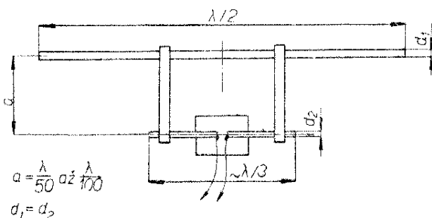
Obr. 18. Transformace T
