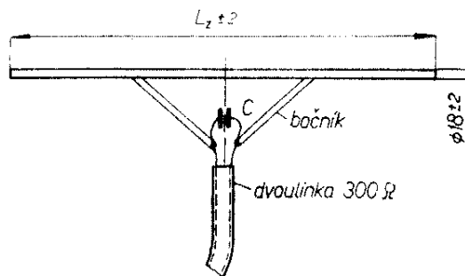
Obr. 54. Bočníkový dipól
