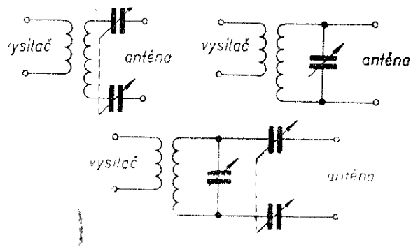
Obr. 96. Připojení antény typu Zeppelin ke koncovému stupni vysílače
