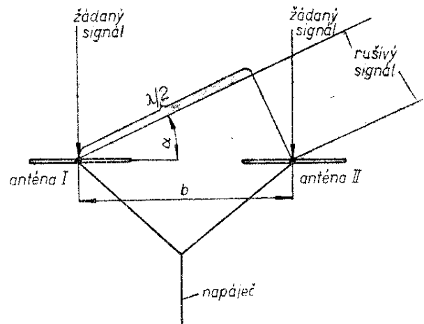
Obr. 77. Potlačení rušivého signálu použitím dvou antén
