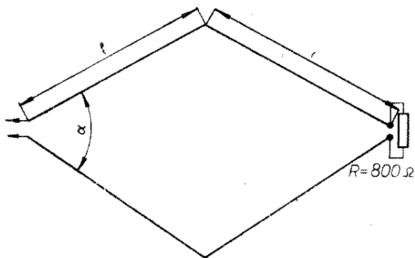
Obr. 73. Kosočtverečná anténa
