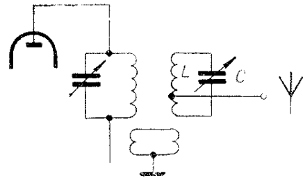
Obr. 82. Připojení antény Windom ke koncovému stupni vysílače
