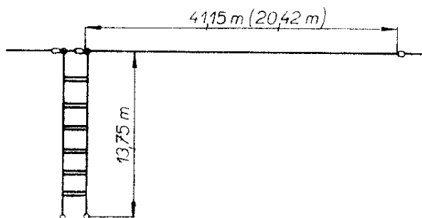
Obr. 97. Anténa typu Zeppelin pro všechna pásma
