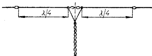
Obr. 87. Půlvlenný dipól napájený zkroucenou linkou
