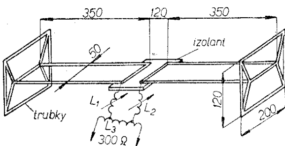
Obr. 47. „Minianténa“ pro I. televizní pásmo
