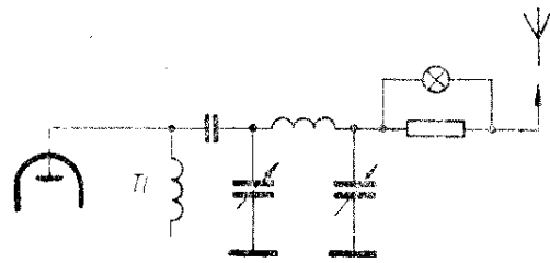
Obr. 123. Indikace anténního proudu žárovkou
