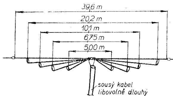
Obr. 110. Anténa pro všechna pásma napájená sousým kabelem
