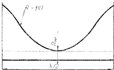
Obr. 17. Průběh reálné části impedance půlvlnného dipólu
