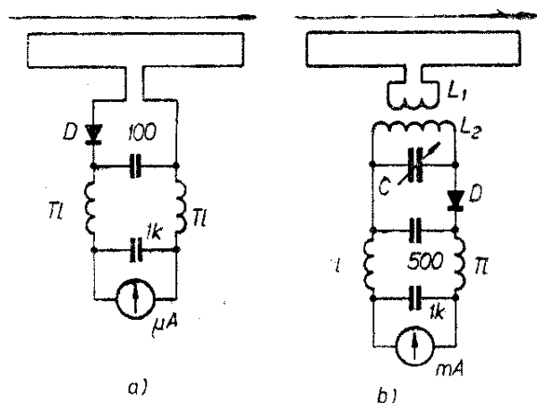
Obr. 129. Přístroje pro měření stojatých vln
