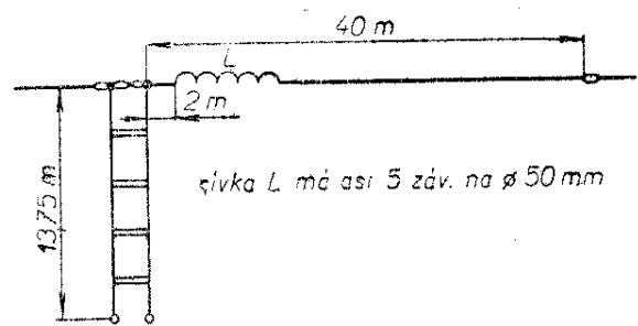
Obr. 93. Anténa DL7AB
