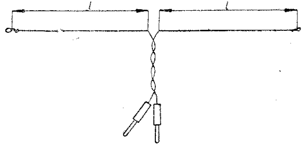
Obr. 44. Provizorní dipól
