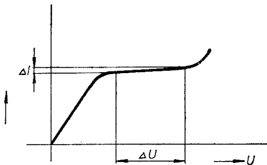
Obr. 3. Charakteristika variátoru
