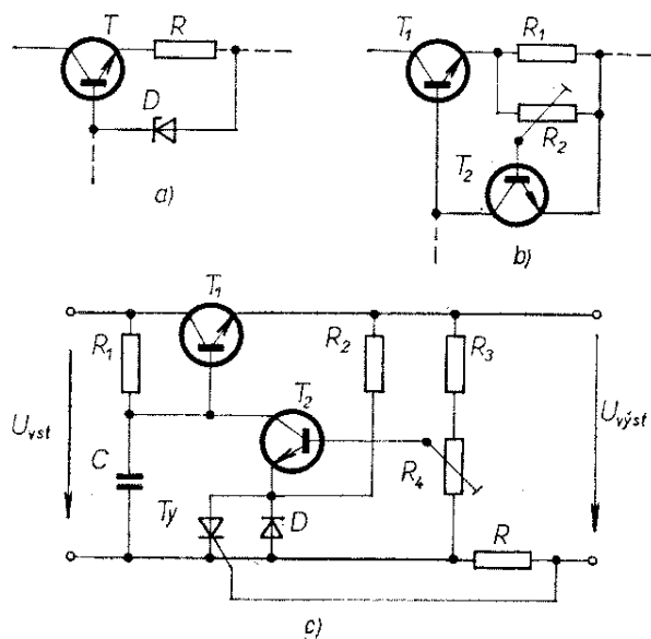
Obr. 65. Elektronická pojistka
