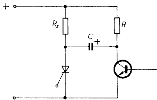
Obr. 44. Vypínání tyristorem
