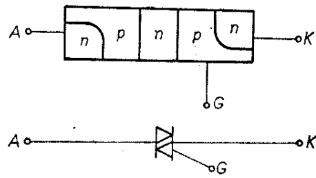
Obr. 46. Triak
