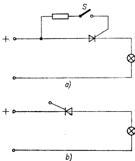
Obr. 45. Zkoušení tyristoru
