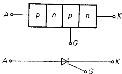
Obr. 38. Tyristor
