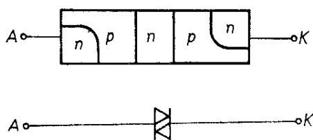
Obr. 48. Diak
