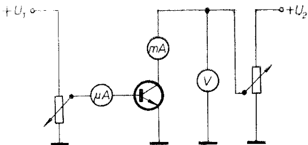
Obr. 35. Měření tranzistorů
