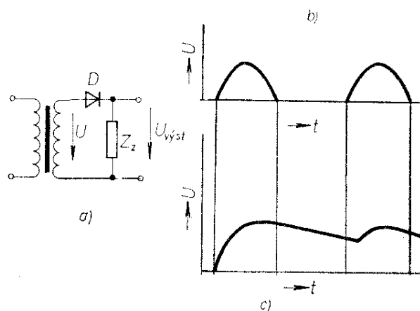
Obr. 51. Jednocestný usměrňovač
