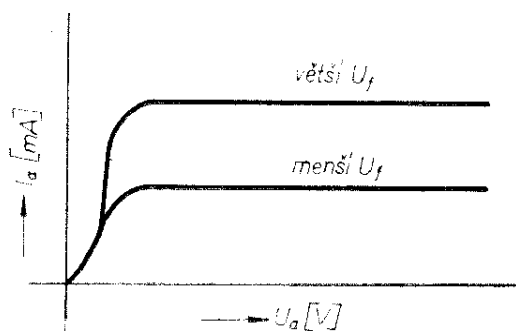
Obr. 17. Anodová charakteristika
